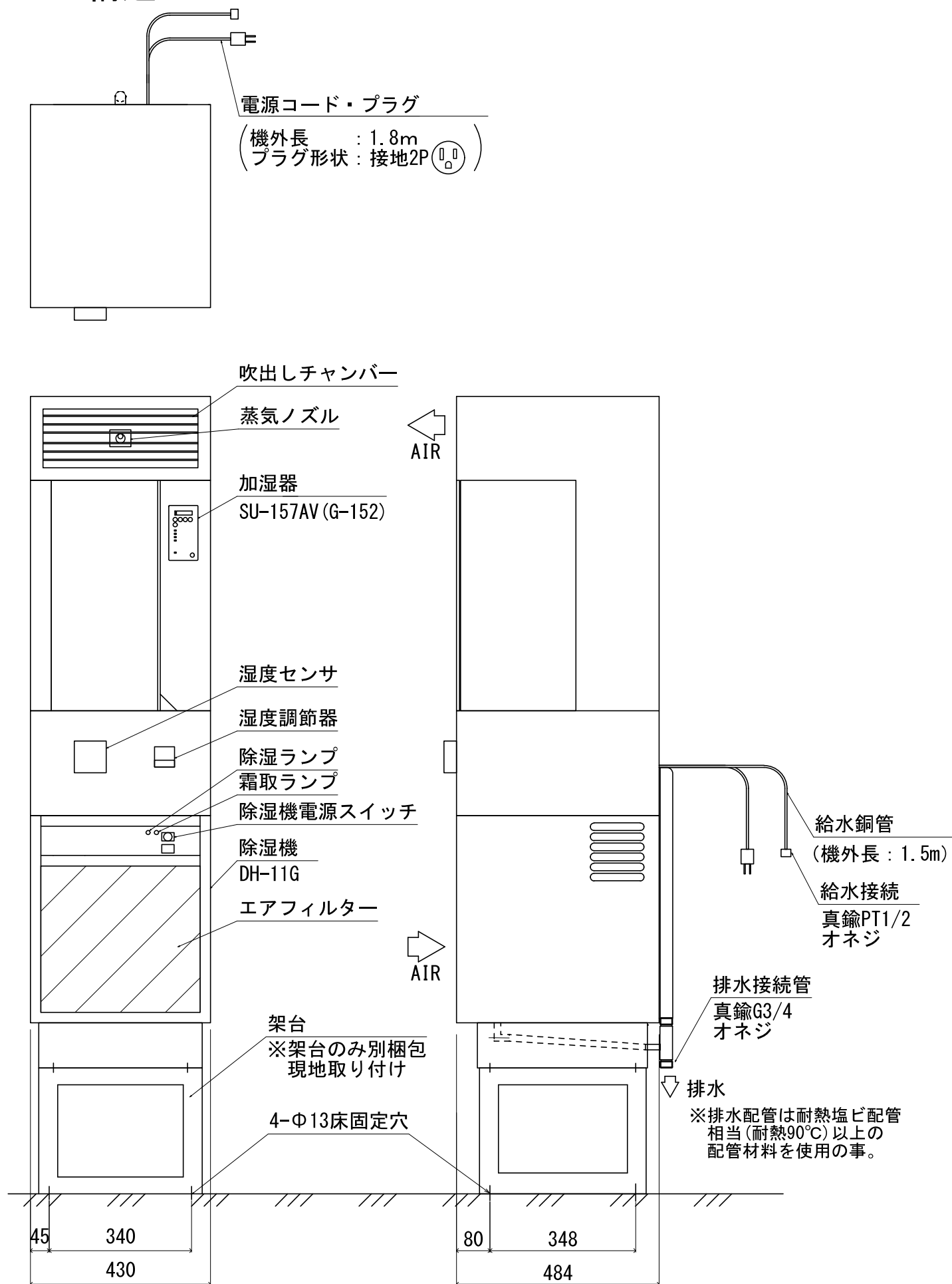
(図3-1 G-152構造図)
