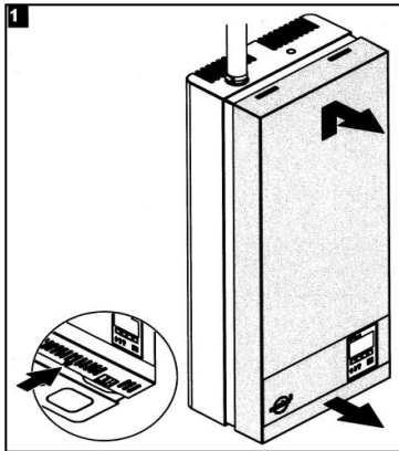
1. 手動排水にてシリンダー内の水を全排水します。 底面のネジを緩め、前面カバーを外します。
