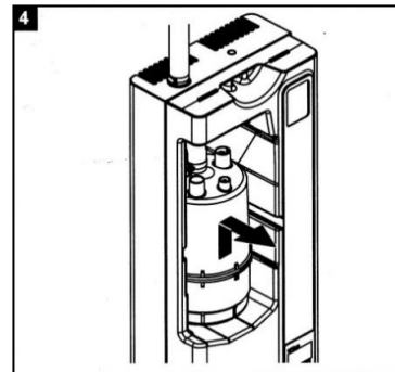
4. 蒸気シリンダーを上引き抜き、外します。 新しい蒸気シリンダーを逆の手順で設置してください。
