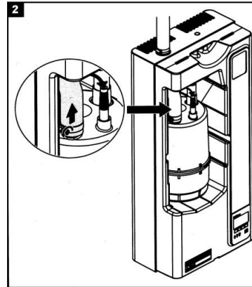
2. 蒸気ホースのバンドを緩め、蒸気ホースを外します。
