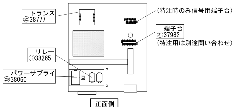
A-A' 断面図 (G-403制御部)
