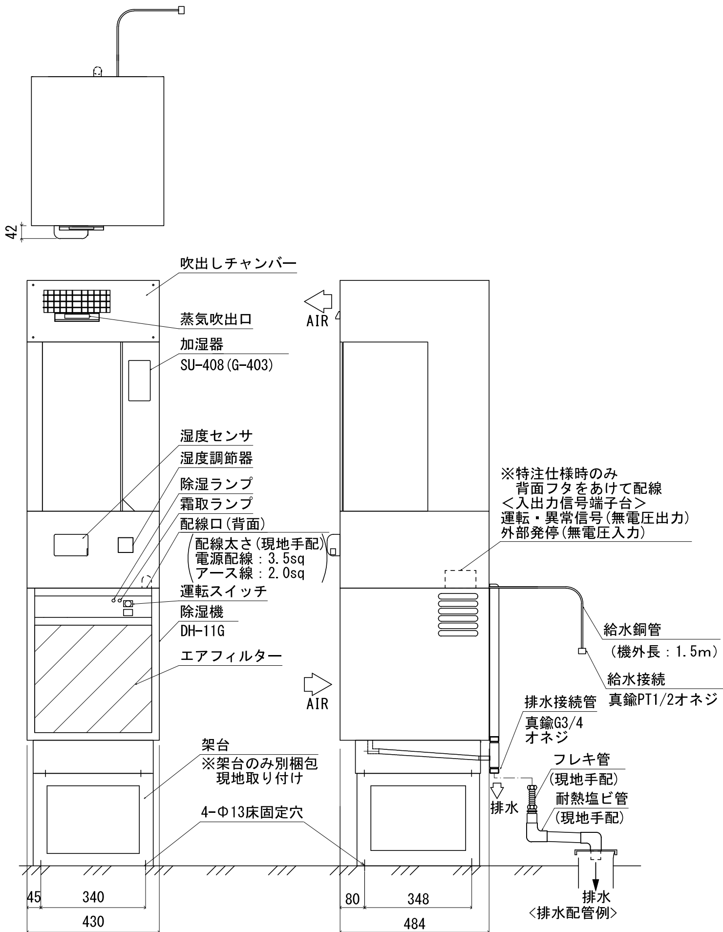
(図3-1 G-403構造図)
