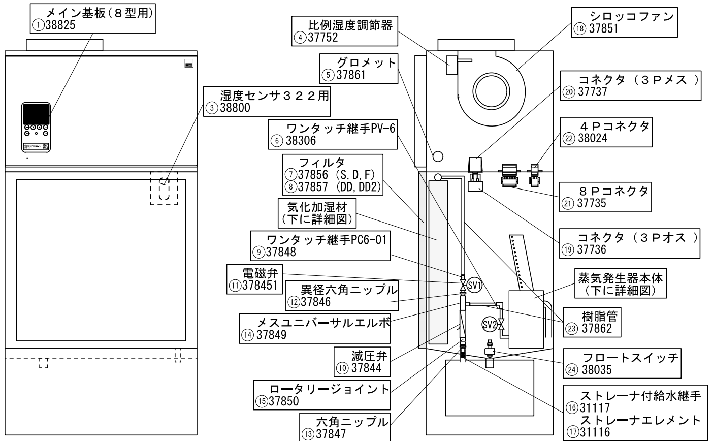
<NES-322D正面図>
