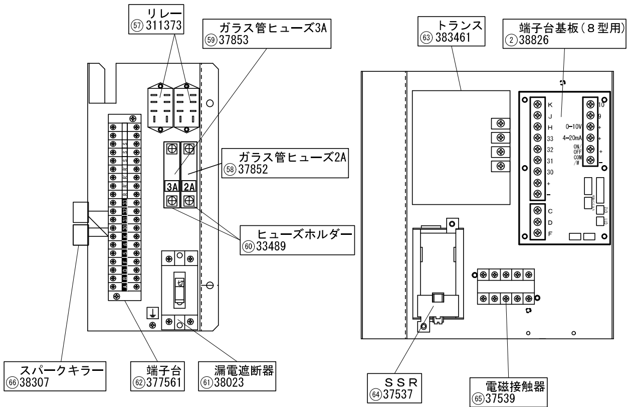
<電装部正面>
