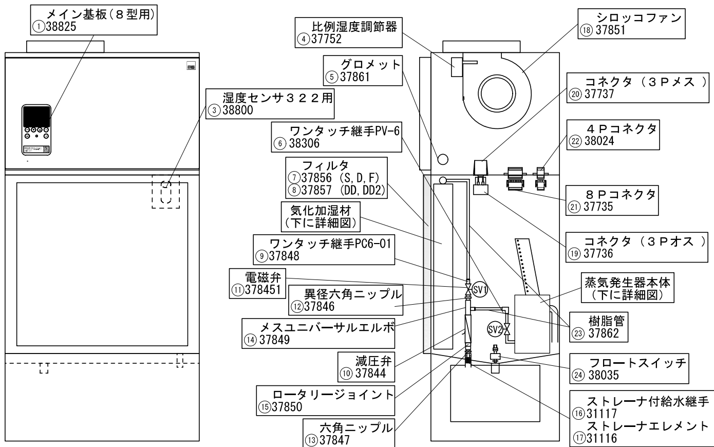
<NES-322D正面図>
