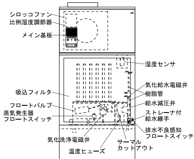
(図6-1 NES-322構造)
